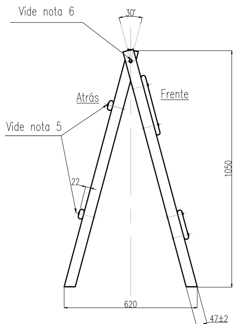
Tipo II : Frente com tábuas e atrás com ripas.
