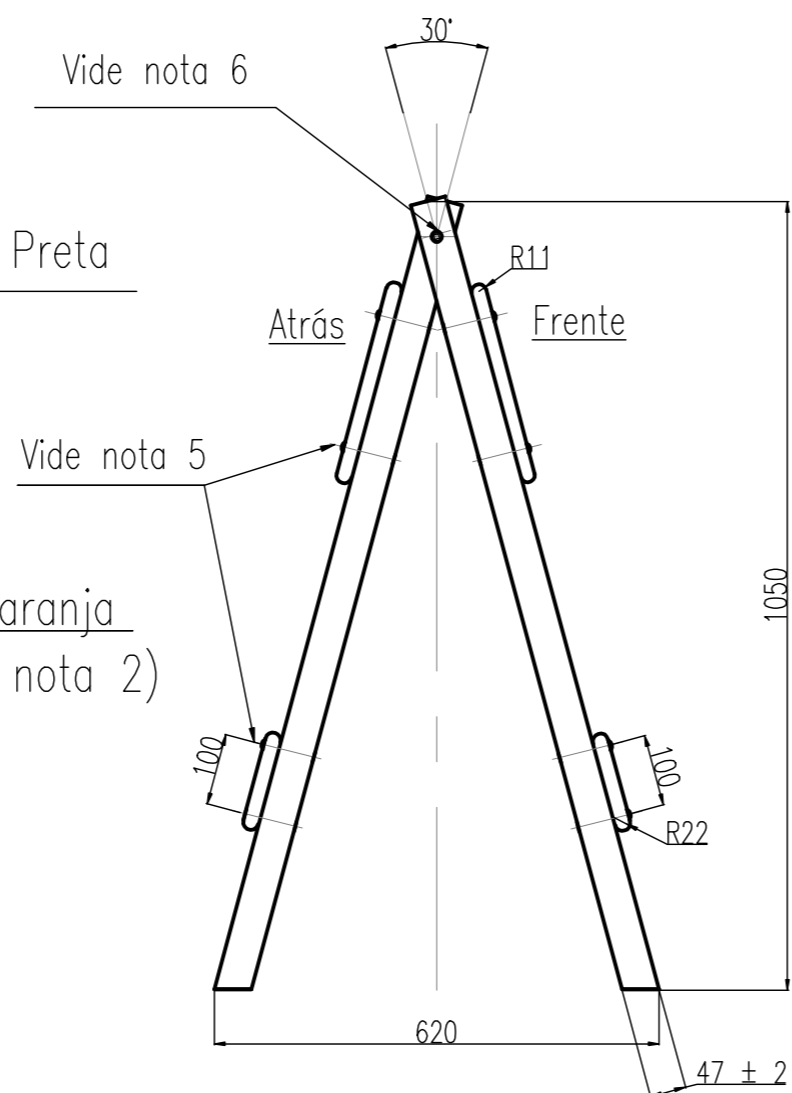
Tipo I : Frente e atrás iguais com tábuas.
